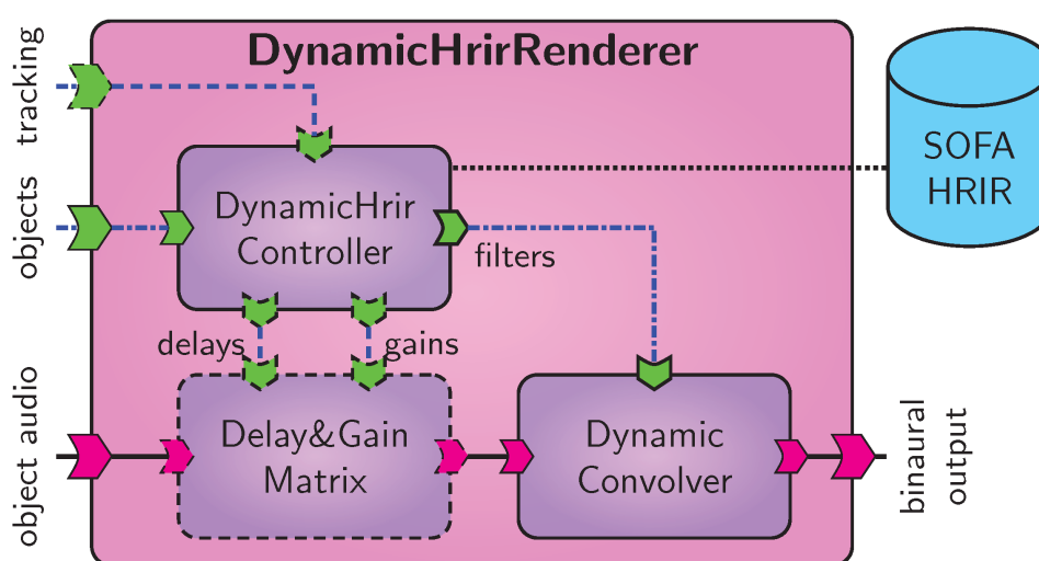
Fig. 10: DynamicHrirRenderer component
